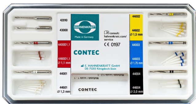
Pivoti Din Fibra De Sticla Hahnenkratt Contec set
